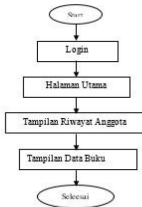
Gambar 3 Flowchart Sistem Usulan pada Anggota
