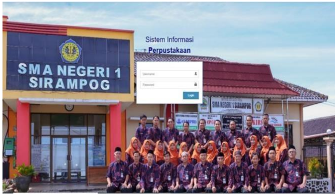
Gambar 12 Halaman Login
